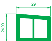
4405 Thermal Insert For 4005, 4006, 4007 cill
